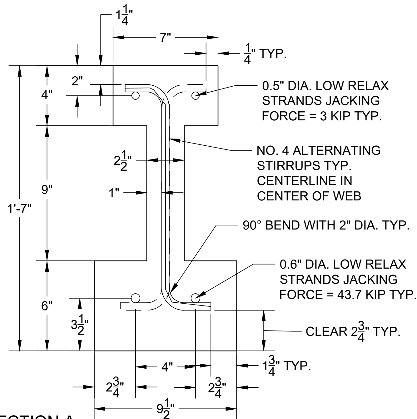
1 SECTION A SCALE: 1" = 3"
